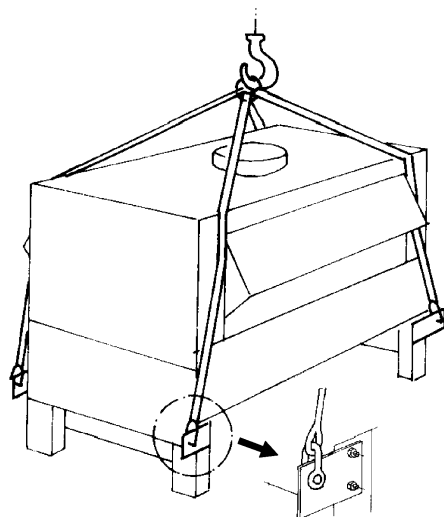
Рис. 12 Подъем
