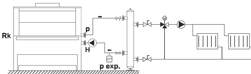
Рис. 18 Пример гидравлической системы
