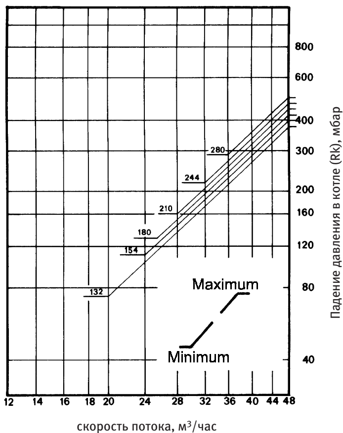
Рис. 19 Объем воды:
