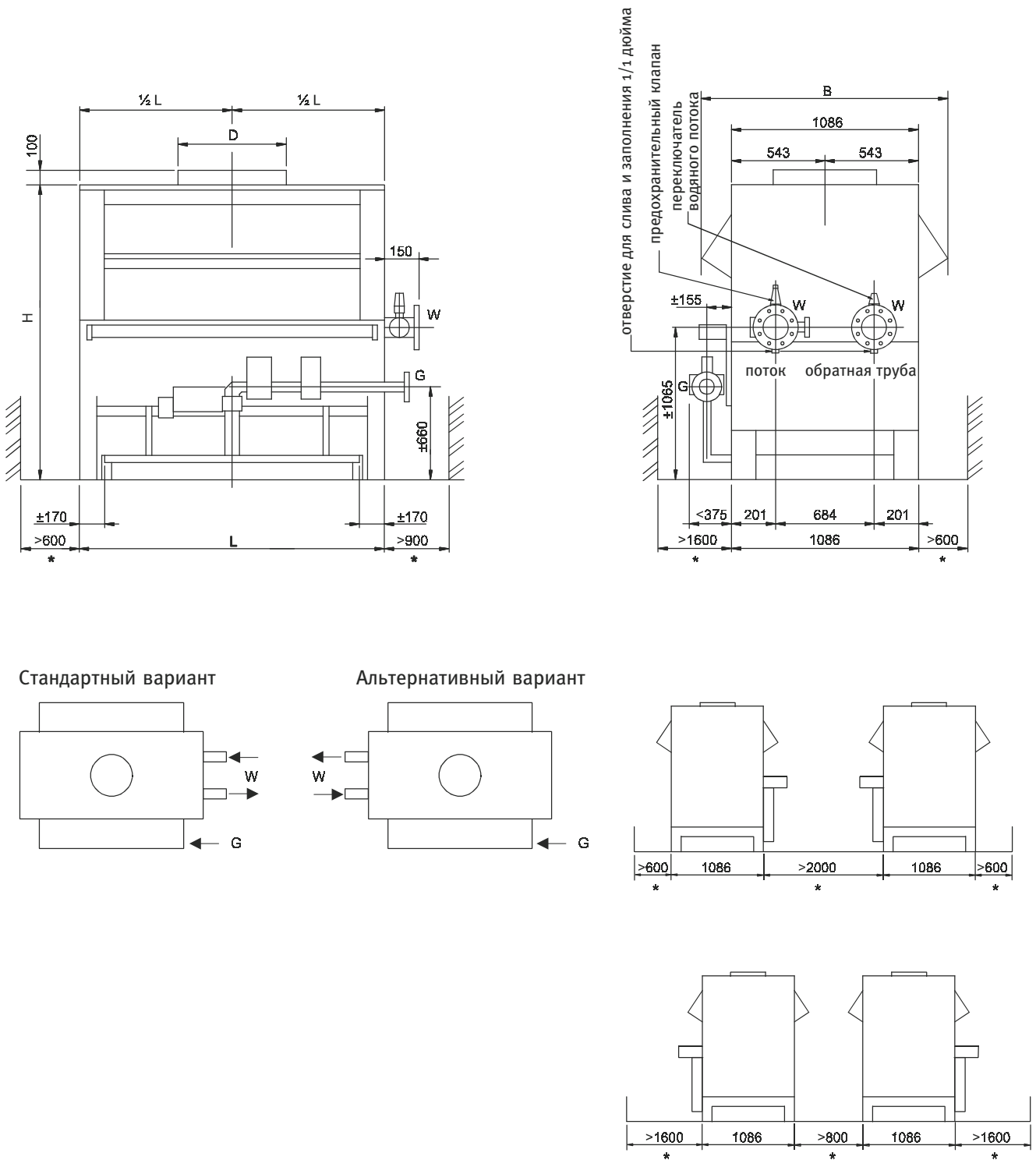
Рис. 1 Габаритные размеры
