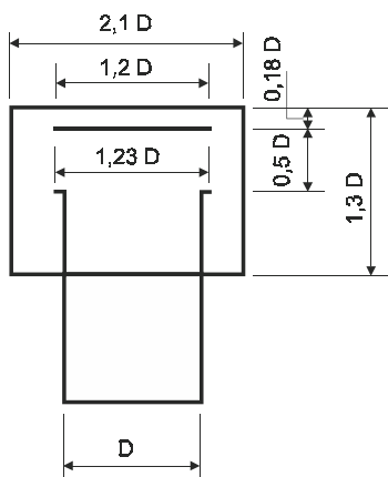
Рис. 16 Оголовье выпуска
