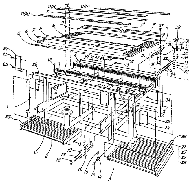
Рис. 7 Горелка
