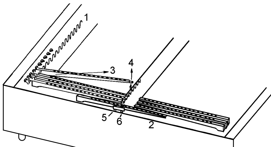
Рис. 31 Узел горелки
