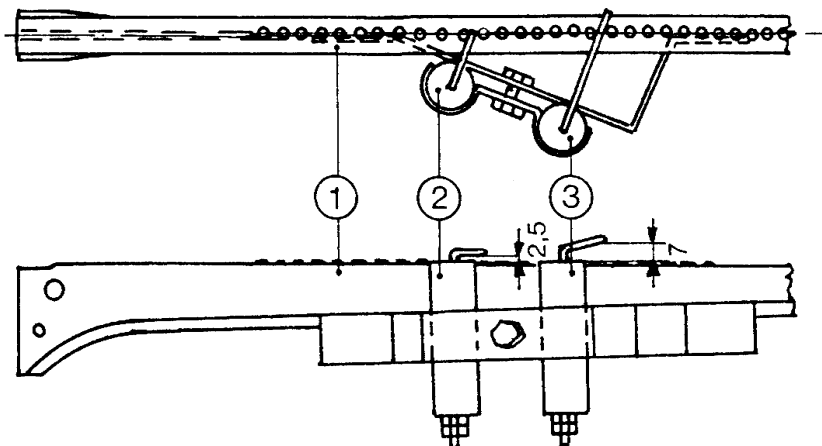
Рис. 32 Электроды
